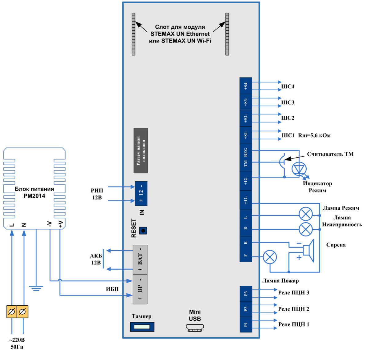
Рис. 11.2. Схема внешних подключений контроллера
