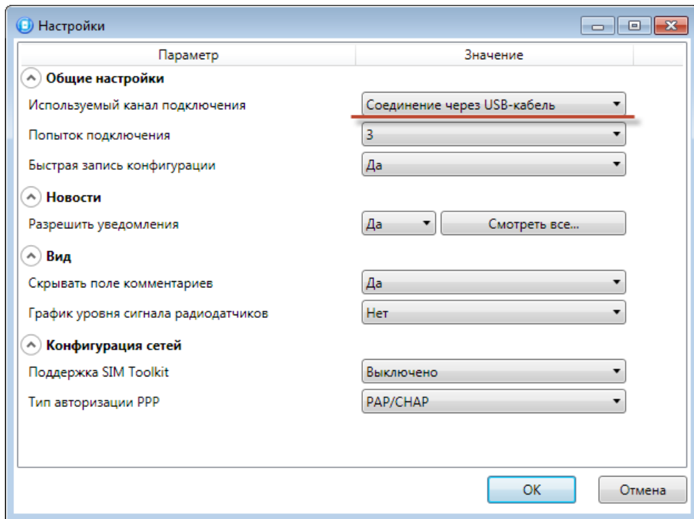
Рис. 4.6. Окно Настройки
