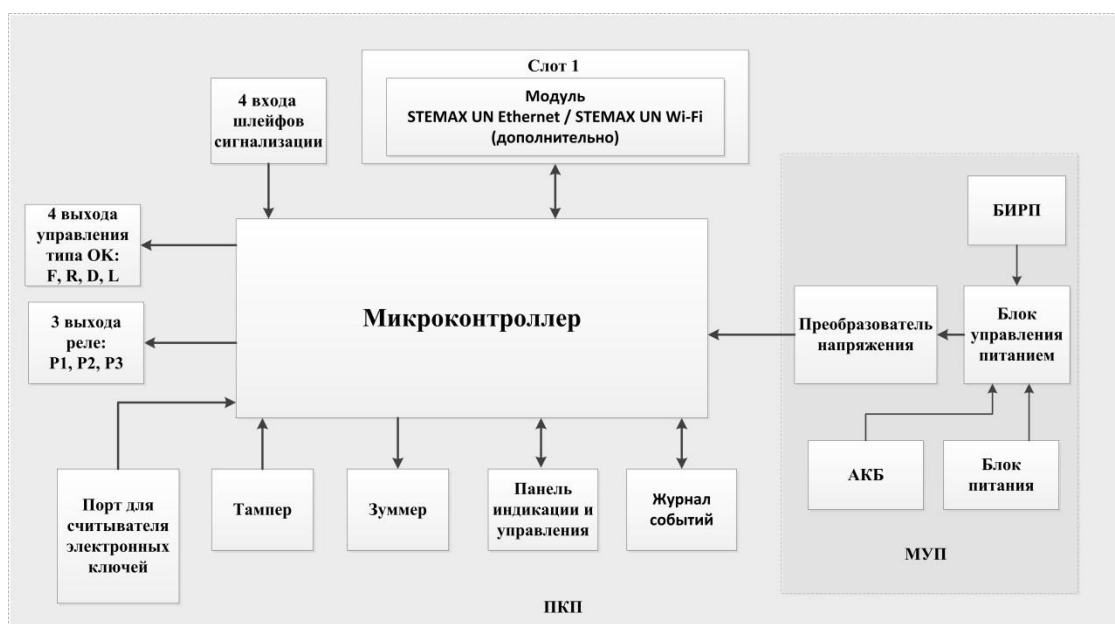
Рис. 3.1. Функциональная схема
